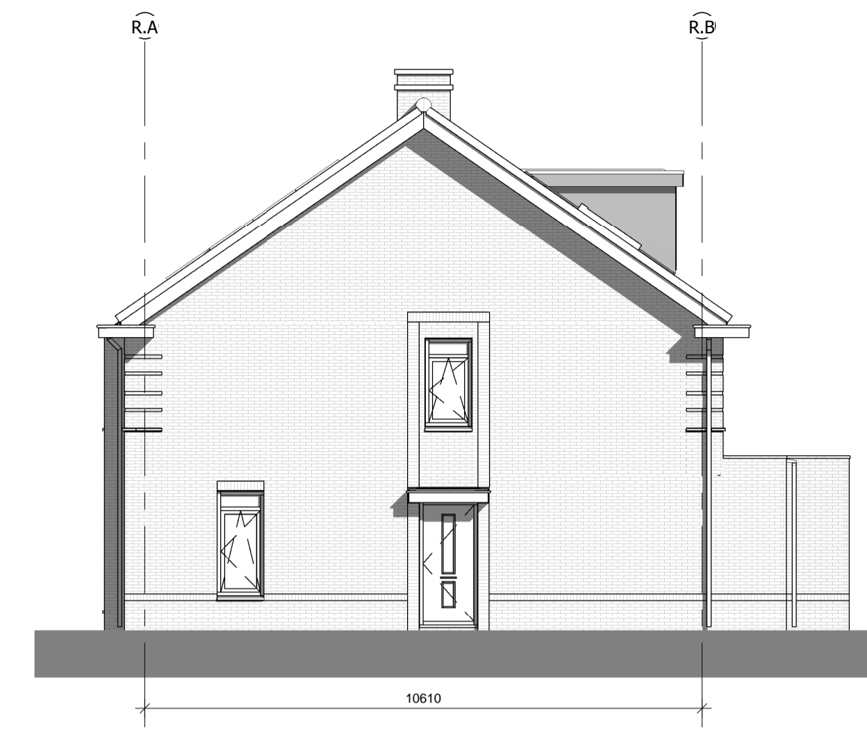
rechter zijgevel
