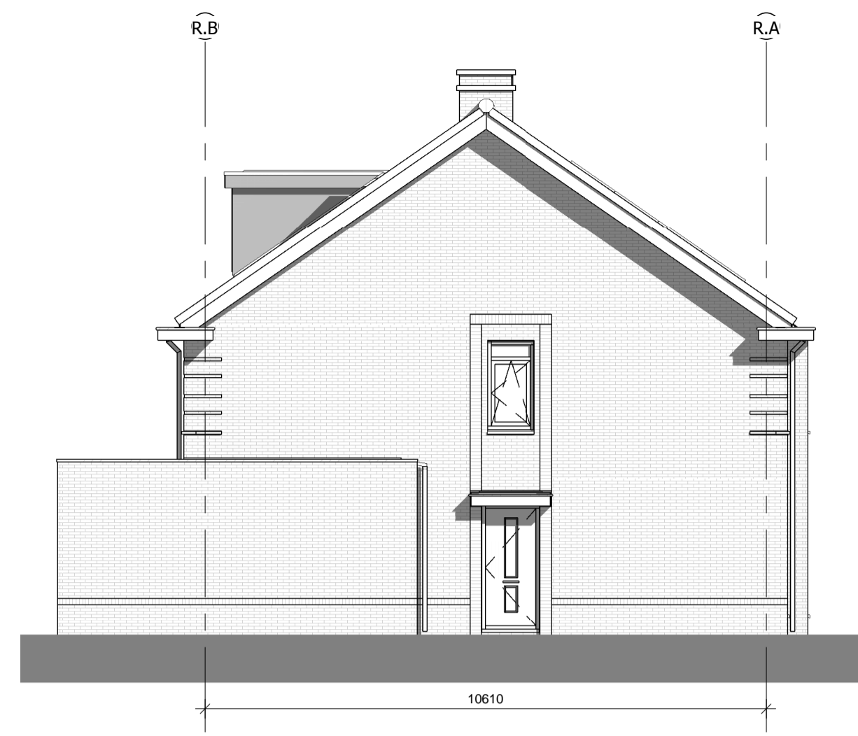
linker zijgevel
